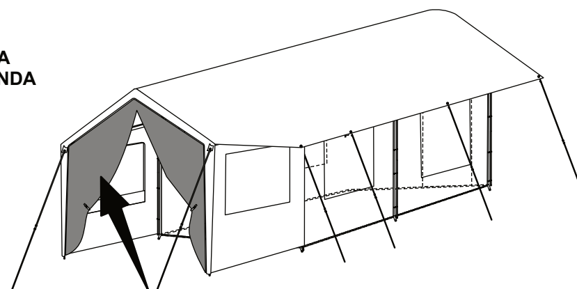
VERANDA FRONT WALL MUR AVANT DE VÉRANDA PAREDE FRONTAL DA VARANDA
